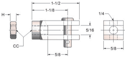
SM-45 ROD CLEVIS, NUT & PIN
